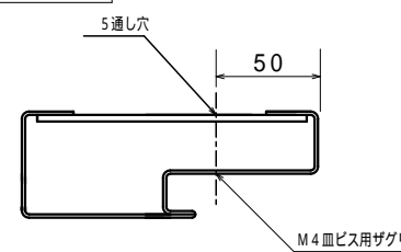
扉枠ビス穴位置
