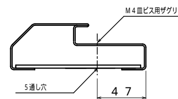
扉枠下部答摺り枠ビス穴位置
