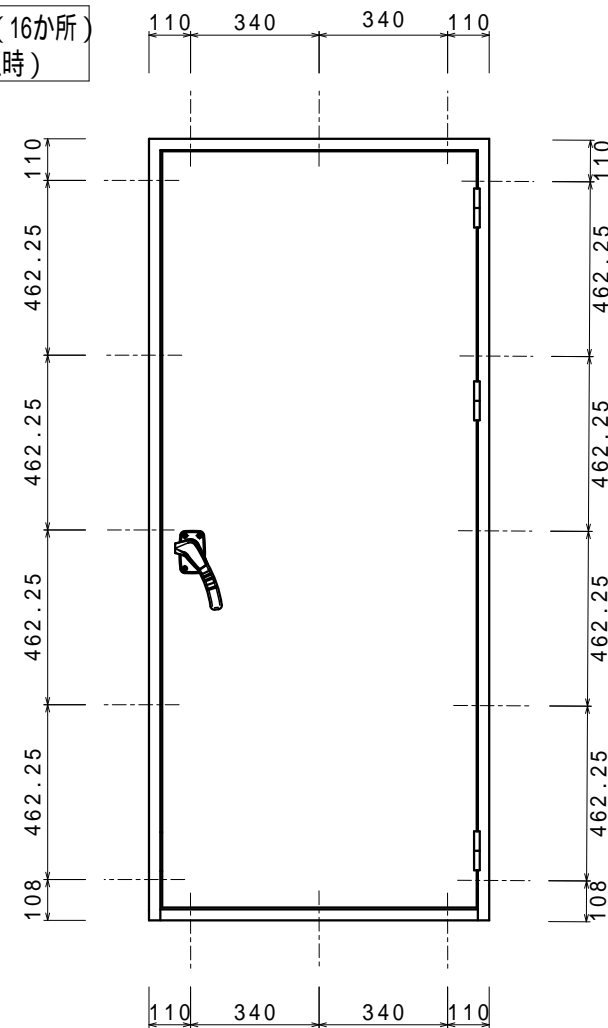
扉枠下部答摺り枠ビス穴位置
